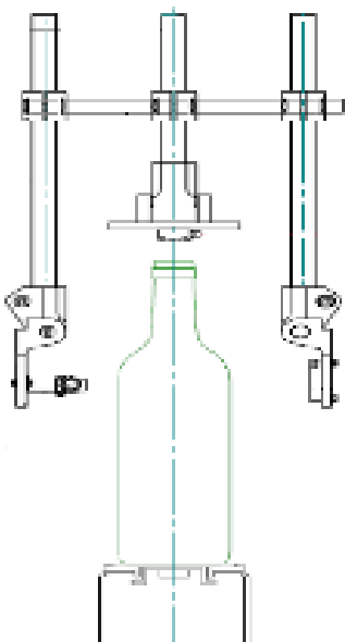
VISTA FRONTALE
